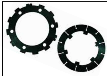
REF. 91243 JUEGO DISCOS EMBRAGUE METÁLICOS MONTESA COTA 348
