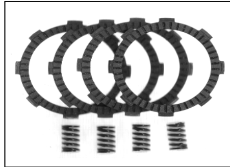
REF. 07613 KIT EMBRAGUE HONDA NSR-MTX COMETICIÓN
